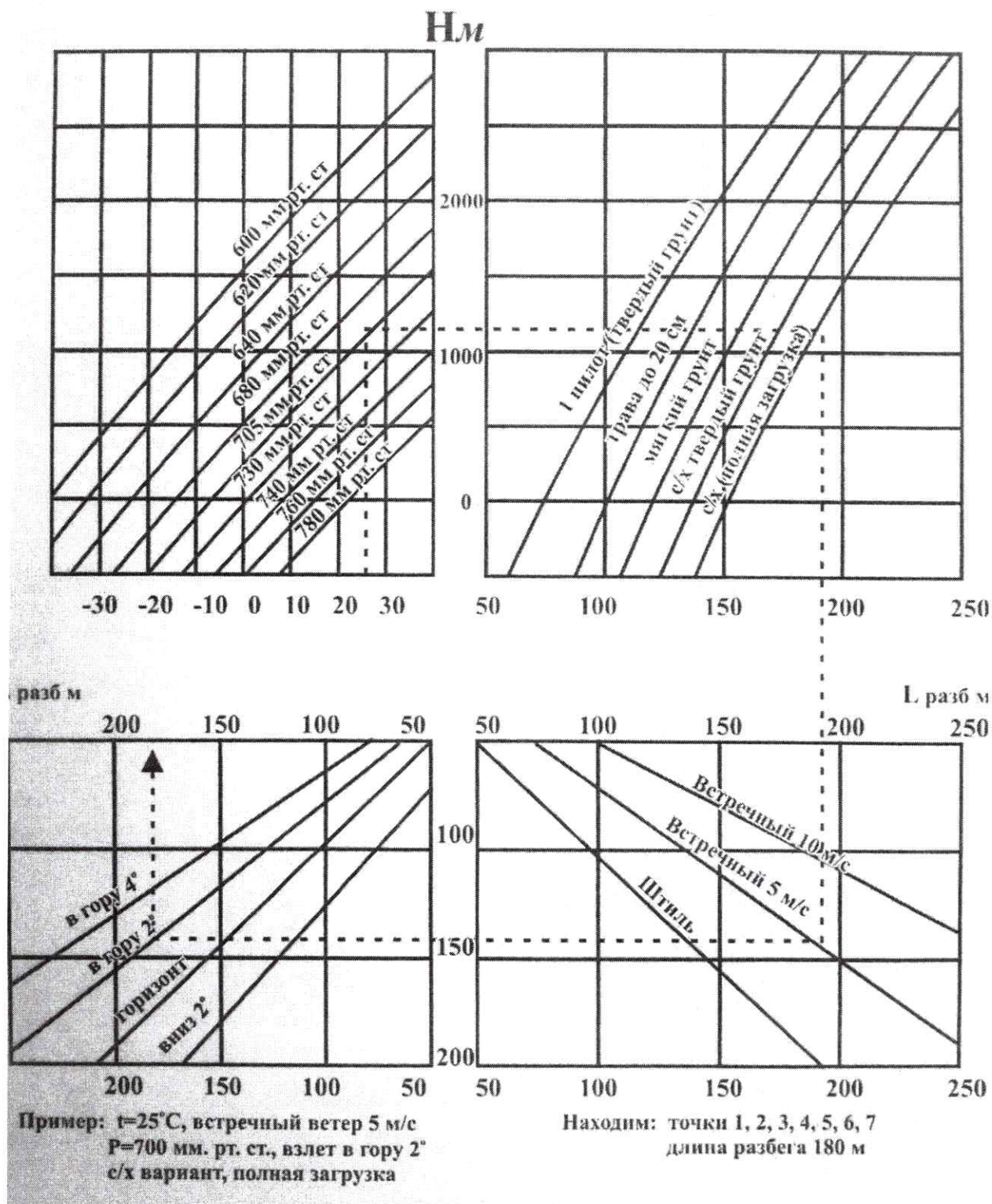
График для определения длины разбега самолета F-02 в зависимости от давления, температуры, скорости ветра и угла площадки
